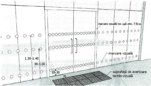
Fig. V.24. – Exemplu de conformare a suprafețelor vitrate în cadrul foi de uși și realizarea contrastului vizual, atunci când ușa și suprafețele adiacente sunt vitrate
