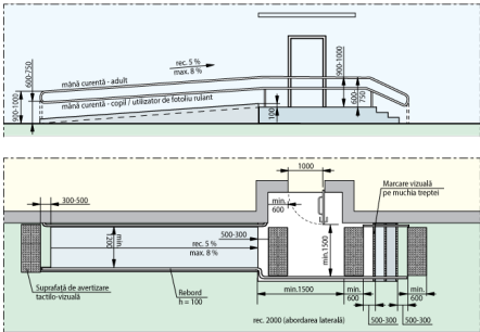
Fig. V.32.b Pămi de acces paralelă cu intrare în clădire
