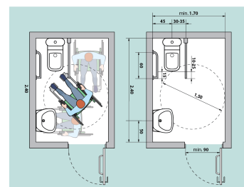
Fig. V.42.a Amplasarea unei cabine WC adaptate - tip B
