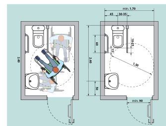
Fig. V.42.b Amenajarea unei cabinete WC adaptate - tip B
