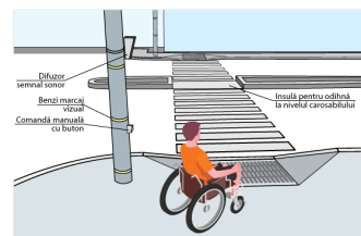
Fig. IV.14.a Traversarea străzii cu lățime mai mare pe 4 benzi de circulație. Perspectivă
