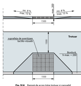
Fig. IV.8 Rampă de acces între trotuar și carosabil
