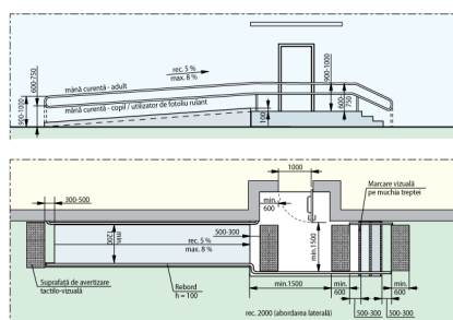
Fig. V.32.2 Rampă de acces paralelă cu intrarea în clădire
