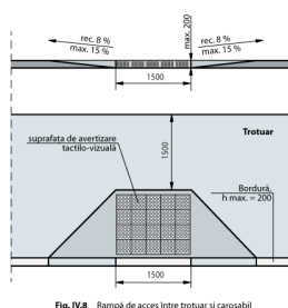
Fig. IV.8 Rămpă de acces între trotuar și carosabil
