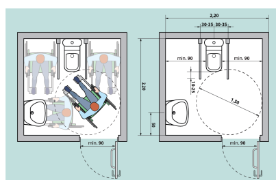
Fig. V42a Aranjarea unei cabine WC adaptate - tip A
