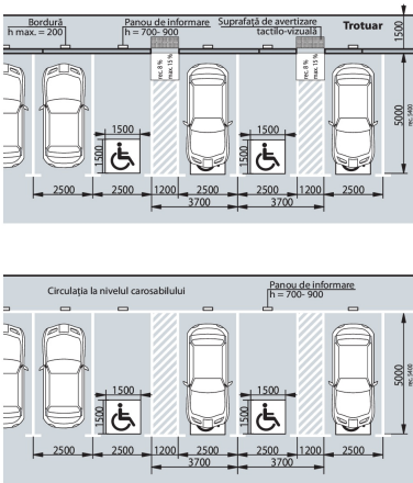
Fig. IV.18 Parkerare pe o direcție perpendiculară față de carosabil
