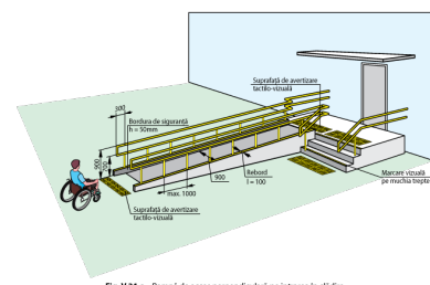
Fig. V.31.a Rampă de acces perpendicular pe intrarea în clădire
