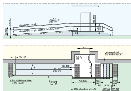
Fig. V.32.b Rampă de acces paralel cu intrarea în clădire
