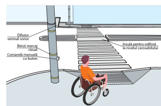
Fig. IV.14.a Traversarea străzii cu lățime mare pe 4 benzi de circulație. Perspectivă
