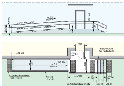
Fig. V.32.b Pampă de acces paralelă cu intrarea în clădire
