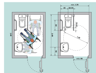
Fig. V42b Amenajarea unei cabine WC adaptate - tip B
