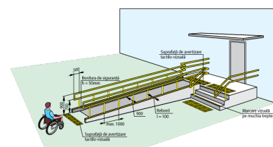
Fig. V.31.a Rampă de acces perpendiculară pe intrarea în clădire
