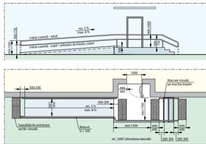
Fig. V.32.b Panta de acces paralelă cu intrare în clădire
