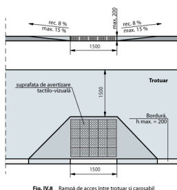
Fig. IV.8 Ramplă de acces între trotuar și carosabil
