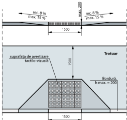
Fig. IV.8 Rampă de acces între trotuar și carosabil
