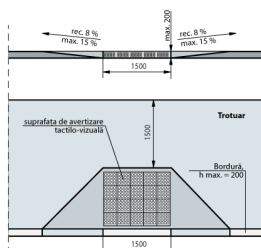
Fig. IV.8 Ramă de acces între trotuar și carosabil
