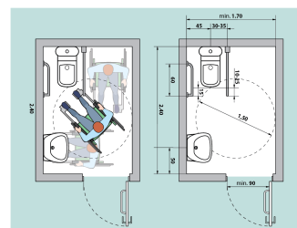
Fig. V.41.a Amenajarea unei cabine WC adaptate - tip B
