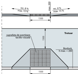
Fig. IV.8 Rămpă de acces între trotuar și carosabil
