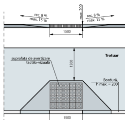
Fig. IV.8 Rampe de acces între trotuar și carosabil
