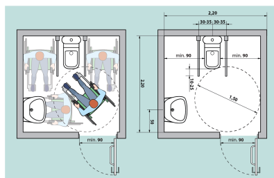
Fig. V.42.a Amplasarea unei cabină WC adaptate - tip A
