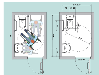
Fig. V.43.a Amplasarea unei cabină WC adaptate - tip B
