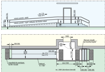
Fig. V.32.b Rampă de acces paralelă cu intrarea în clădire
