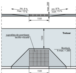
Fig. IV.8 Ramplă de acces între trotuar și carosabil
