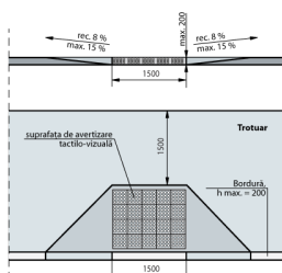
Fig. IV.3 Rampă de acces între trotuar și carosabil
