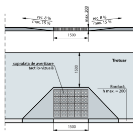
Fig. IV.8 Ramplă de acces între trotuar și carosabil
