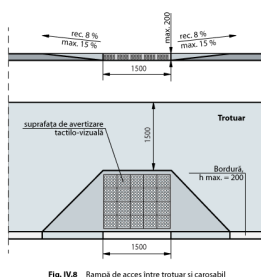
Fig. IV.8 Ramplă de acces între trotuar și carosabil
