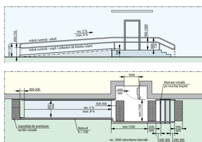
Fig. V.32.b Rampă de acces paralelă la intrare în clădire
