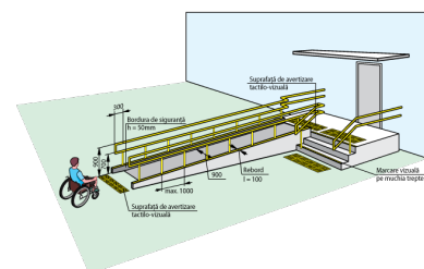
Fig. V.31.a Rampă de acces perpendiculară la intrare în clădire
