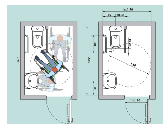
Fig. V.43a Amenajarea unei cabină WC adaptate - tip B
