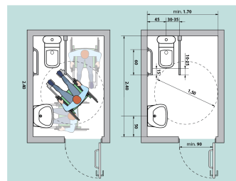
Fig. V.43.a Amenajarea unei cabine WC adaptate - tip I
