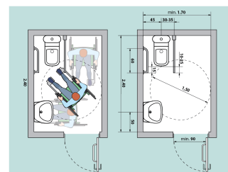
Fig. V43a Aranjarea unei cabine WC adaptate - tip B
