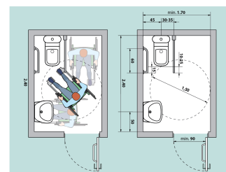
Fig. V42.a Amenajarea unei cabine WC adaptate - tip B
