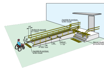
Fig. V.31.a Rămpă de acces perpendiculară pe intrarea în clădire
