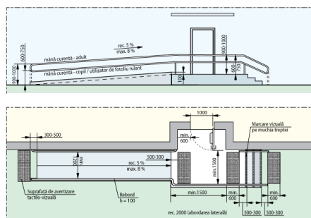
Fig. V.32.b Părpă de acces paralelă cu intrarea în clădire
