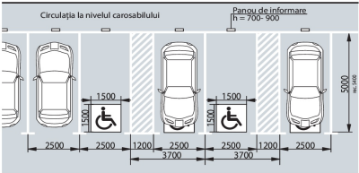
Fig. IV.18 Parcare pe o direcție perpendiculară față de carosabil
