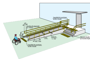
Fig. V.31.a Ramplă de acces perpendiculară pe intrarea în clădire
