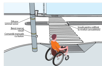
Fig. IV.14.a Traversarea străzilor cu lăţime mai mare de 4 benzi de circulaţie. Perspectivă
