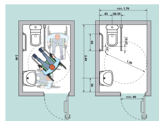
Fig. V.43 a Amplasarea unei cabloze WC adaptate - tip I
