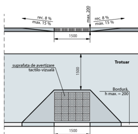
Fig. IV.8 Rampă de acces între trotuar și carosabil
