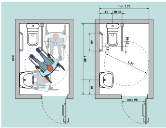
Fig. V.43.b Amenajarea unei cabine WC adaptate - tip B
