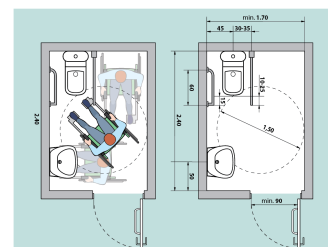
Fig. V43.4 Amenajarea unei cabine WC adaptate - tip B
