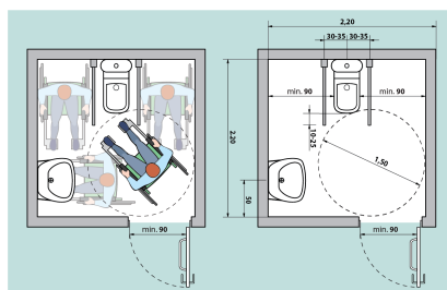
Fig. V42.2 Amenajarea unei cabine WC adaptate - tip A
