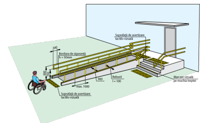
Fig. V.31.a Ramă de acces perpendiculară pe intrarea în clădire
