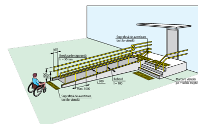
Fig. V.31.a Rampe de acces perpendiculare pe intrare în clădire
