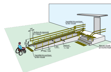
Fig. V.31.1 Rampă de acces perpendiculară pe intrarea în clădire
