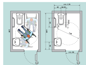
Fig. V42a Amenajarea unei cabine WC adaptate - tip B
