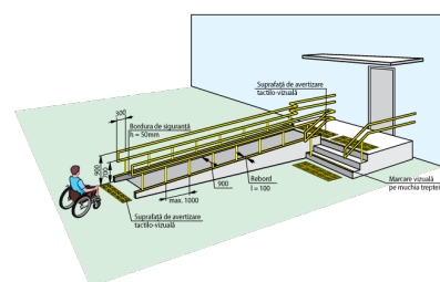
Fig. V.31.a Rampă de acces perpendiculare pe intrarea în clădire
