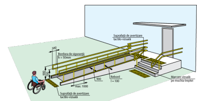
Fig. V.31.a Rampă de acces perpendiculară pe intrarea în clădire
