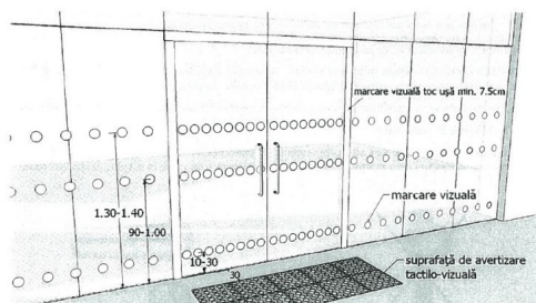
Fig. V.24. - Exemplu de conformare a suprafețelor vitrate în cadrul foilor de ușă și realizarea contrastului vizual, atunci când ușa și suprafețele adiacente sunt vitrate
