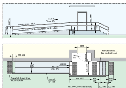
Fig. V.32.b Ramplă de acces paralelă cu intrare în clădire
