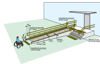
Fig. V.31.a Rampa de acces perpendiculara pe intrarea in cladire
