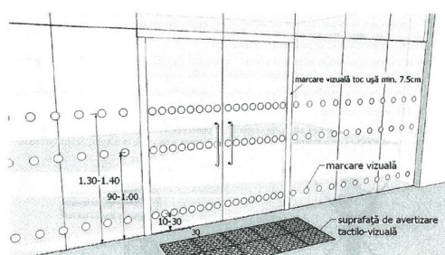
Fig. V.24. - Exemple de conformare a suprafețelor vitrate în cadrul foii de ușă și realizarea contrastului vizual, atunci când ușa și suprafețele adiacente sunt vitrate
