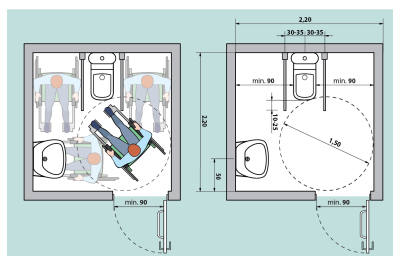
Fig. V.42.1.1. Amplasarea unei cabine WC adaptate - tip A
