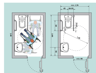
Fig. V42b Aranjarea unei cabine WC adaptate - tip B
