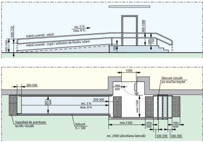
Fig. V.32.b Panta de acces paralelă cu intrarea în clădire
